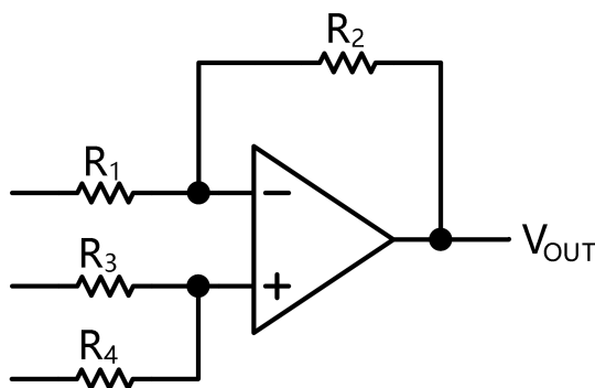
图 4. 差分放大器
