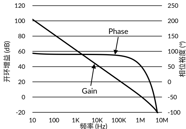
图 11. 开环增益和相位裕度与频率的关系， C_L=100\text{pF}
