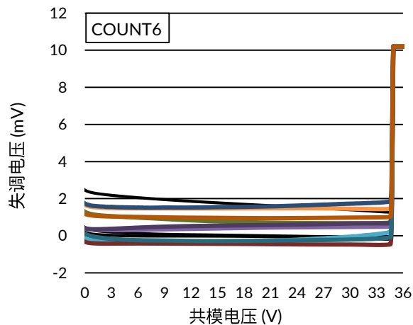
图 3. 失调电压和共模电压的关系
