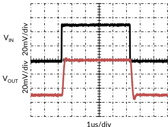
图 7. 50mV 小信号阶跃响应， G=+1 ， C_L=100\text{pF} ， R_L=0
