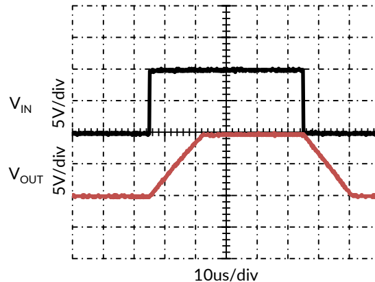
图 8. 10V 大信号阶跃响应， G=+1 ， C_L=100\text{pF} ， R_L=0
