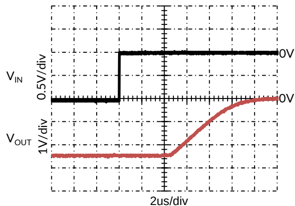
图 10. 反向过载恢复， V_S = \pm 2.5\text{V} ， V_{IN} = 1\text{V } V_{PP} ， G=+11
