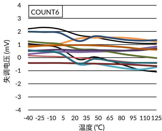
图 4. 失调电压和温度的关系
