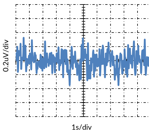
图 6. 0.1Hz~10Hz 输入电压噪声
