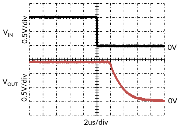
图 9. 正向过载恢复， V_S = \pm 2.5\text{V} ， V_{IN} = 1\text{V } V_{PP} ， G=+11
