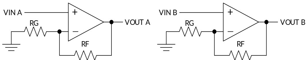
图 13. 应用原理图示意
