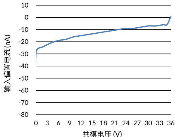
图 5. 输入偏置电流和共模电压的关系
