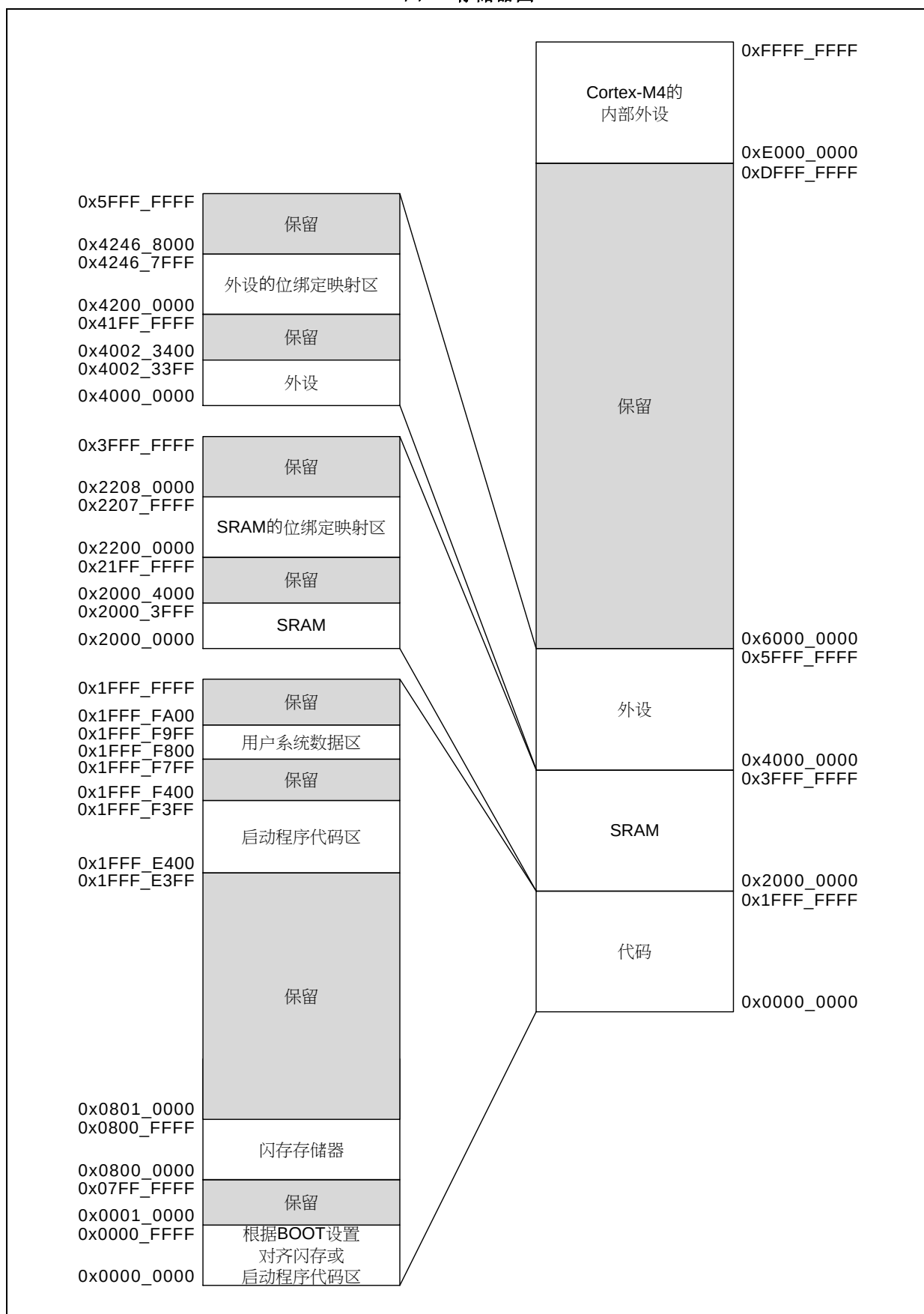
图 7. 存储器图
