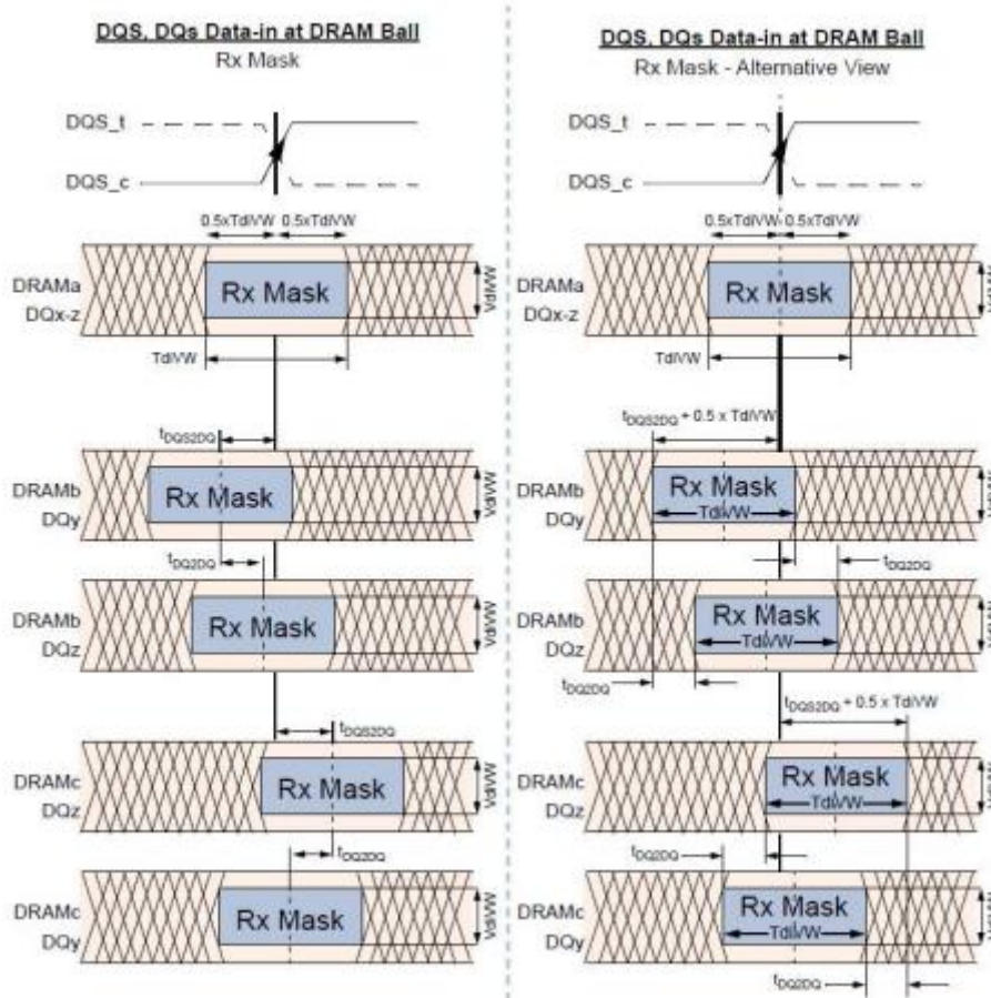
Figure 29 DQS to DQ and DQ to DQ Timings at DRAM Balls
