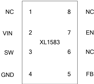
图 2. XL1583 引脚配置
