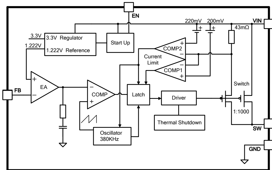
图 3. XL1583 方框图
