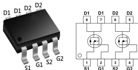
SOP8
