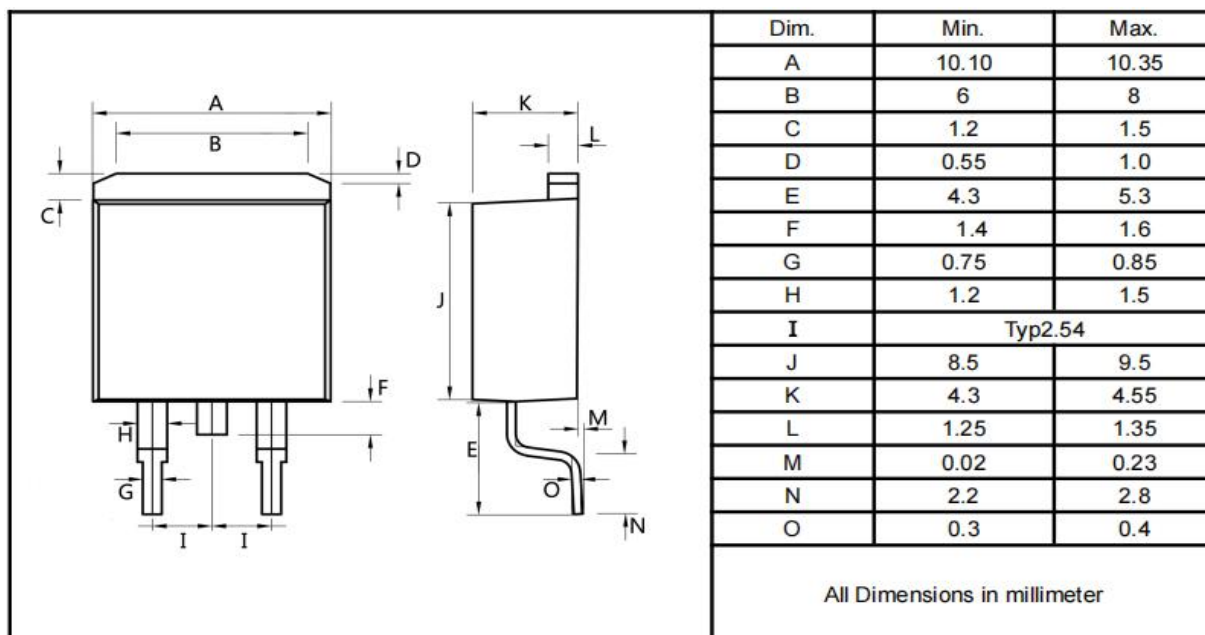
TO-263
