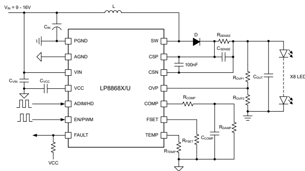
典型升压 LED 驱动器应用原理图
