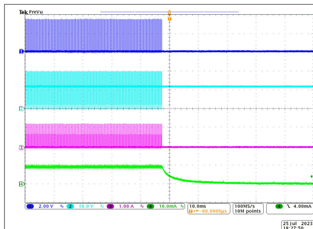
图 8-6. 在 PWM = 1%、4kHz 时关断
