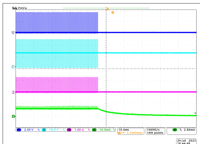
图 8-13. 在 PWM = 1%、4kHz 时关断
