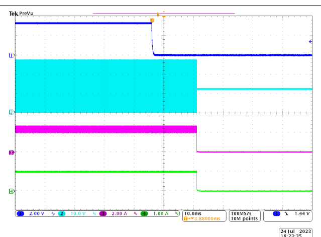
图 8-14. 在 ADIM = 100%、500Hz 时关断
