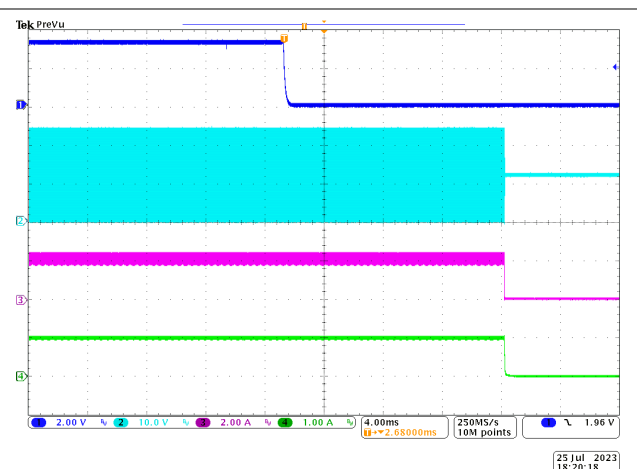
图 8-7. 在 ADIM = 100%、500Hz 时关断
