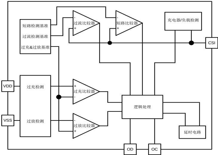
图 3 功能框图
