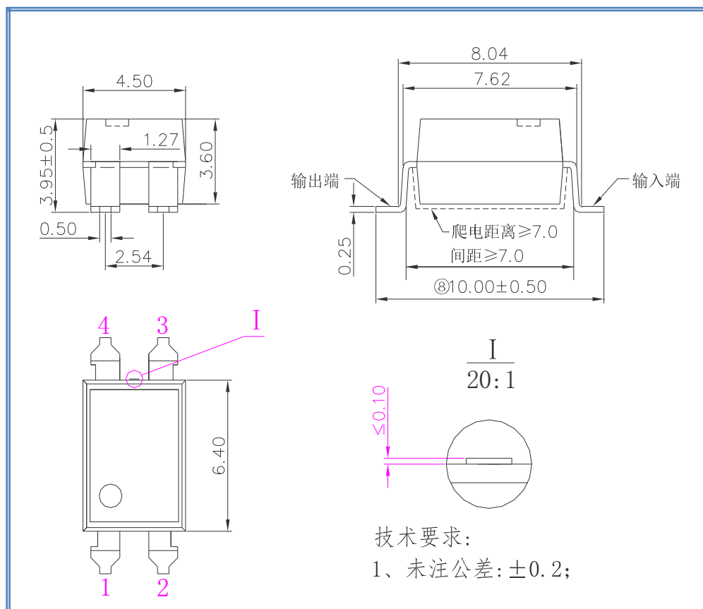
图 4 MT-AQY214EH外形尺寸
