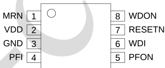
图 2、引脚图
