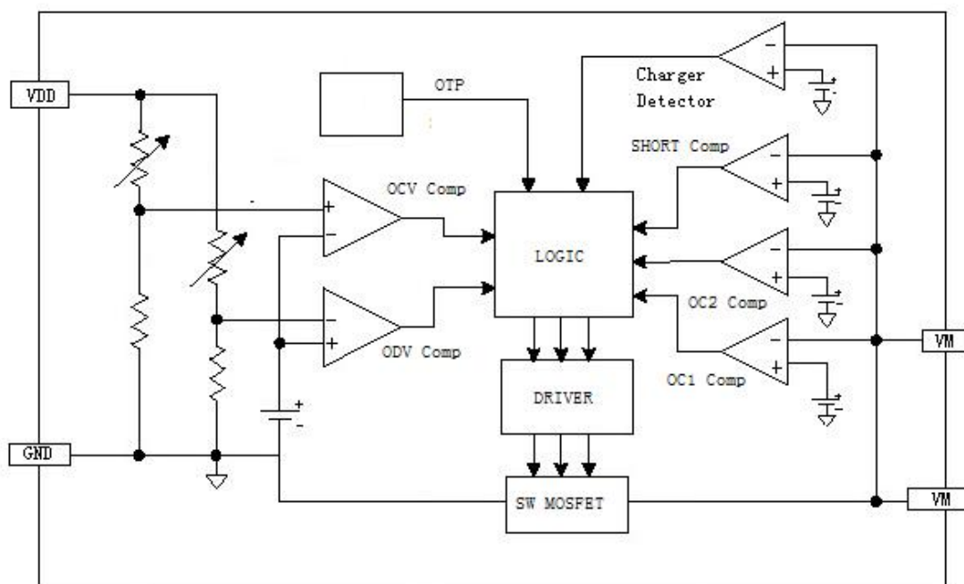
Figure 1. 原理图
