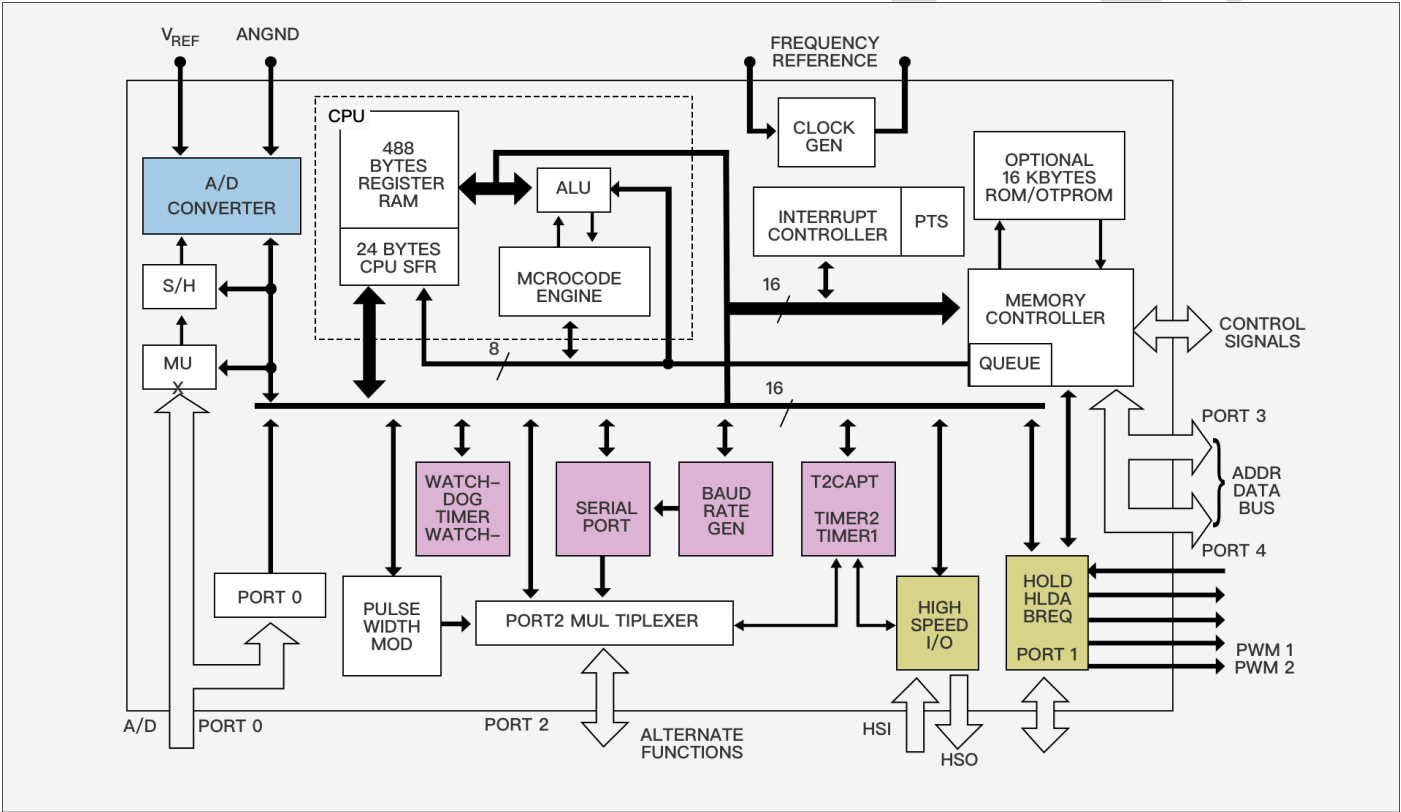
CLM80C196KC20框图
