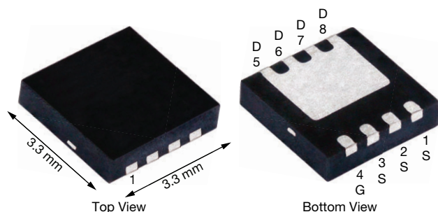
DFN 3x3 EP
