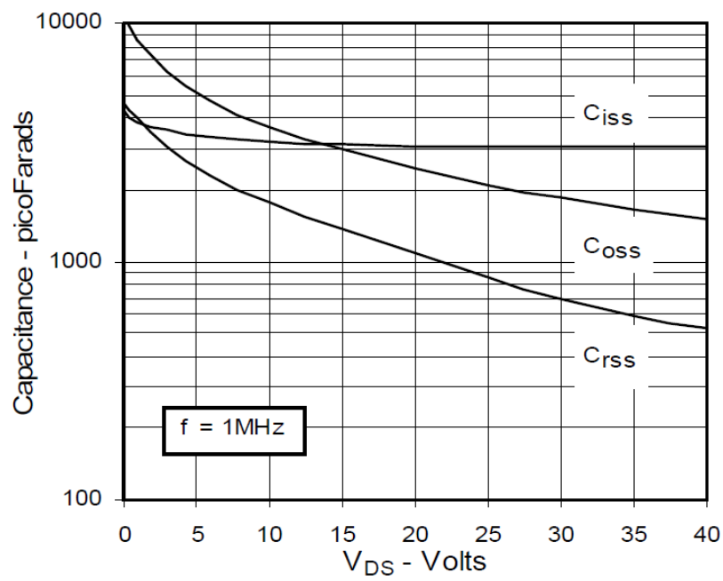
Fig. 11. Capacitance
