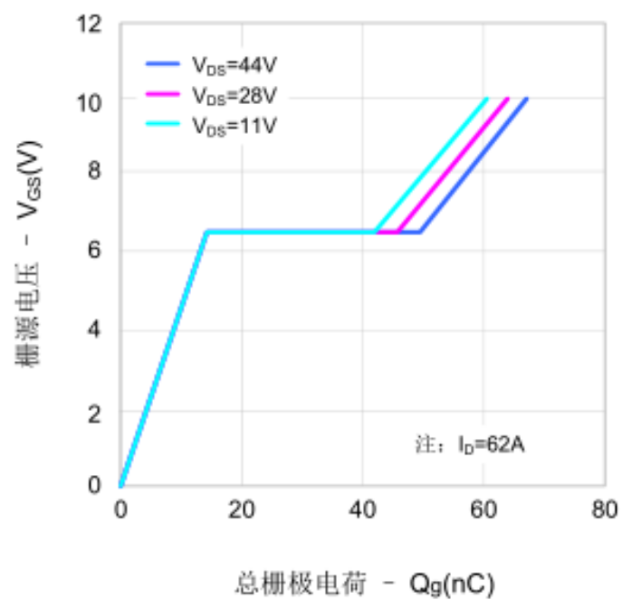
图6. 电荷量特性
