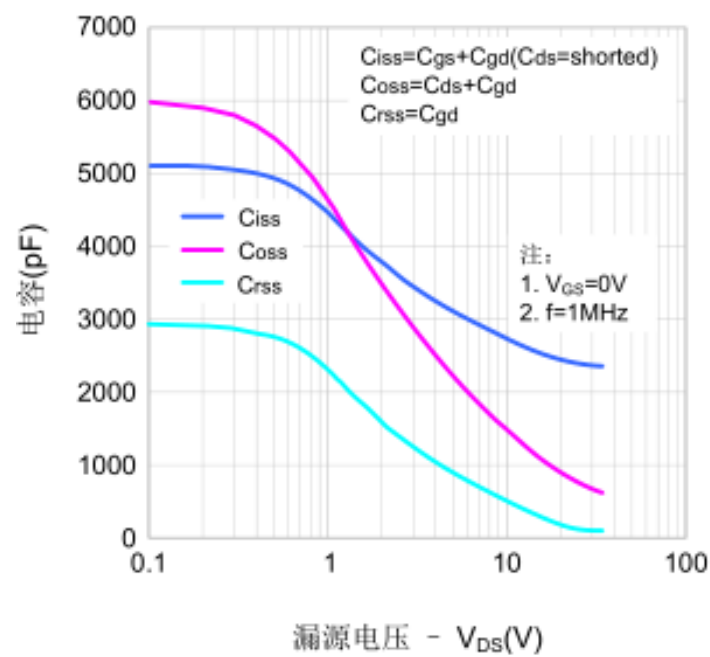
图5. 电容特性
