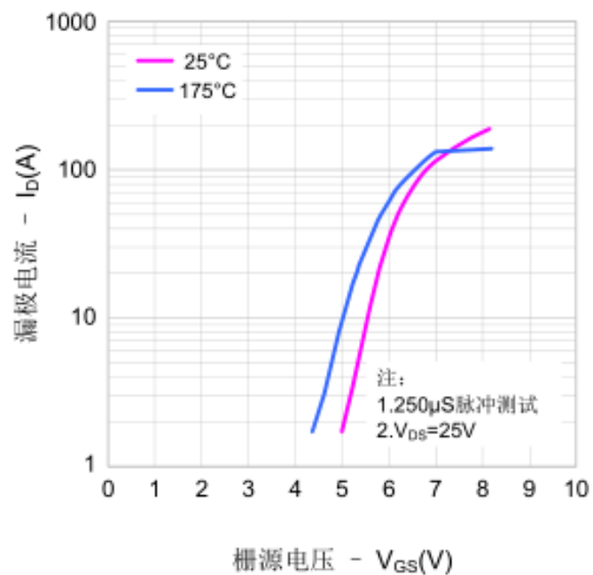
图3. 传输特性
