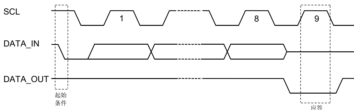
图9 输出应答
