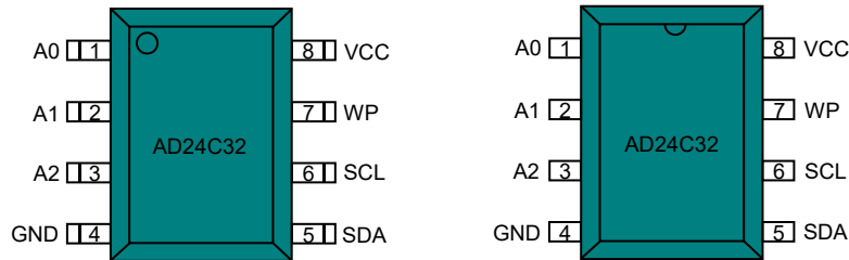
图2 AD24C32引脚定义图
