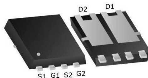
DFN3333-8L
