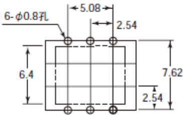
尺寸图(单位:mm)
