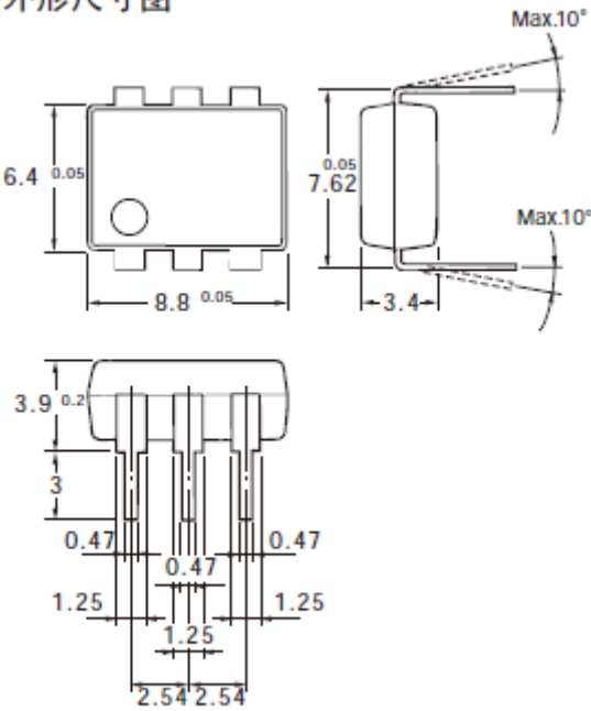
尺寸图(单位:mm)
