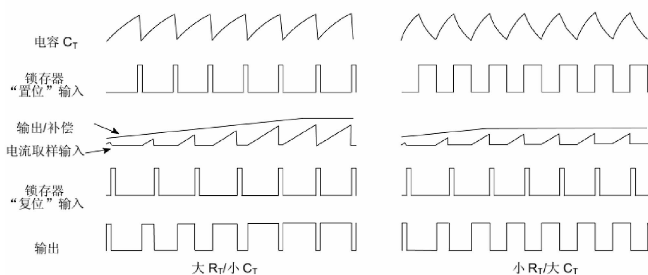
图 18. 时序图
