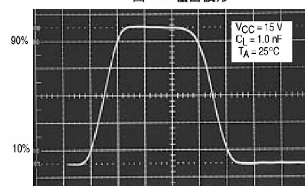
图 14. 输出波形
