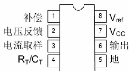
管脚连接图
