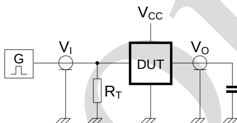
图4 测量开关时间的测试电路
