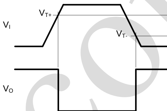
图7 传输特性的定义
