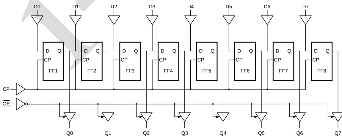
图 3 逻辑框图
