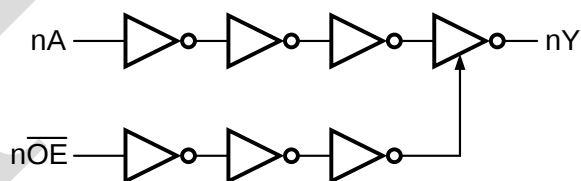
图 3 逻辑框图
