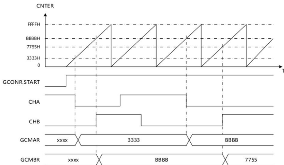
捕获模式示意图
