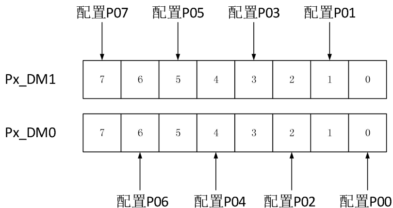
I/O 配置图
