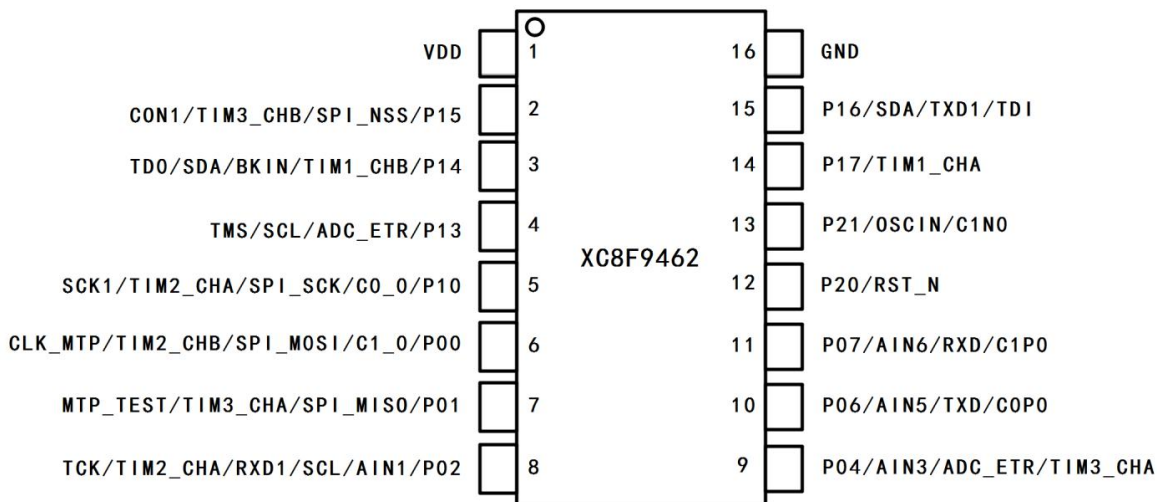
SOP16 封装脚位图
