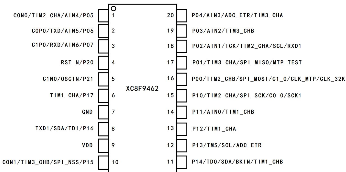
TSSOP20 封装脚位图
