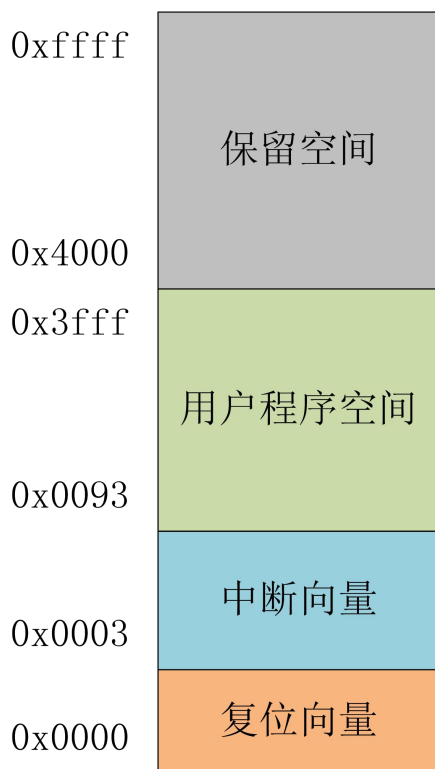
程序存储区结构图
