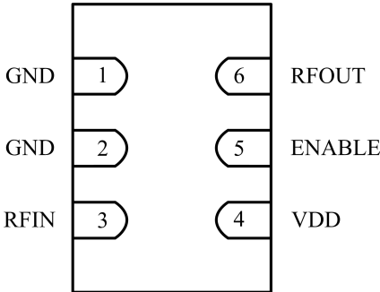
图 2-1 芯片封装管脚排列
