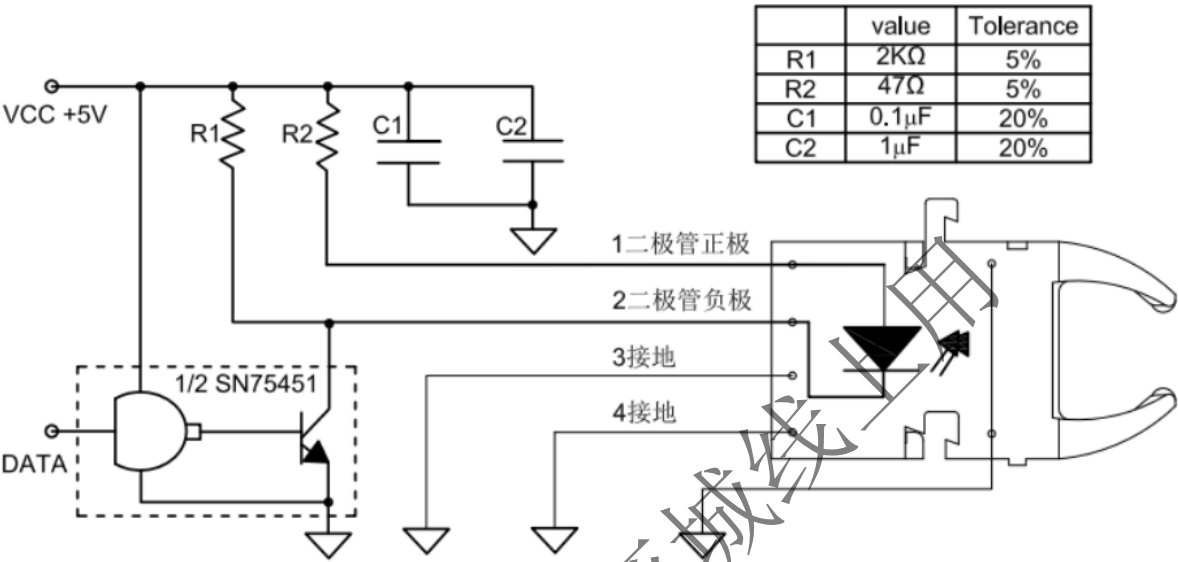
推荐发射的应用线路， V_{cc}=5\text{V}
