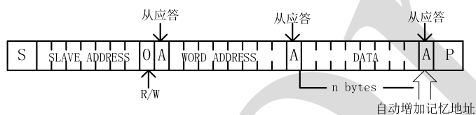
图 9、主传送器到从接收器 (写模式)
