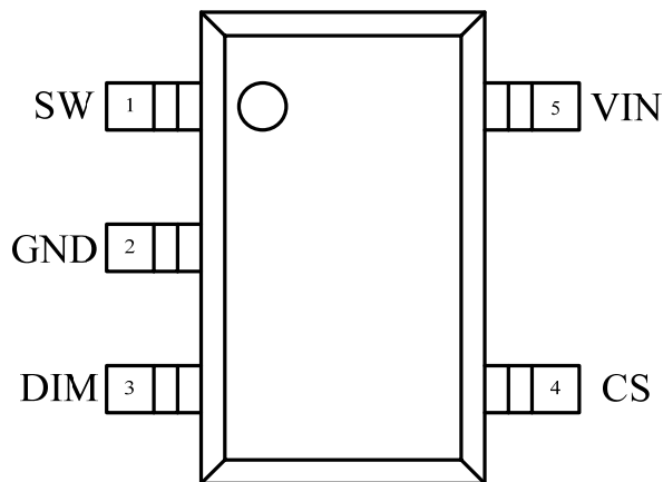
SOT23-5
