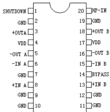
TSSOP20
