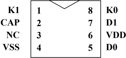
TTP277-AO8N 8-SOP-A
