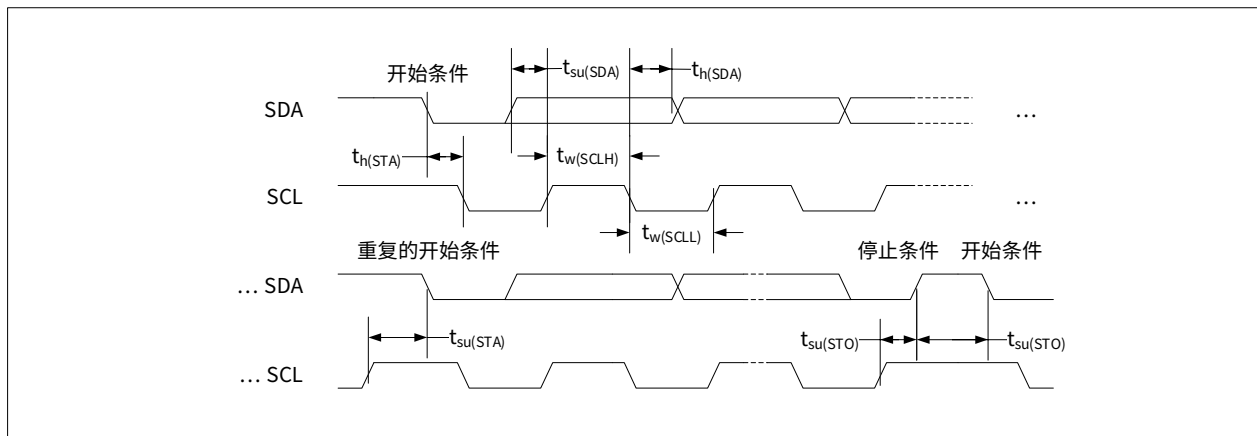
图 7-8 I2C 时序图
