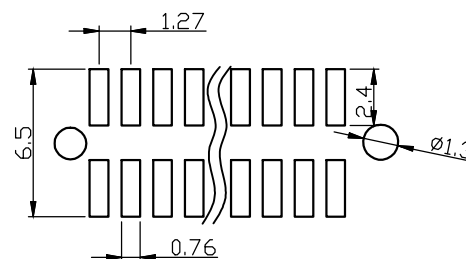
P.C.B Hole Layout
