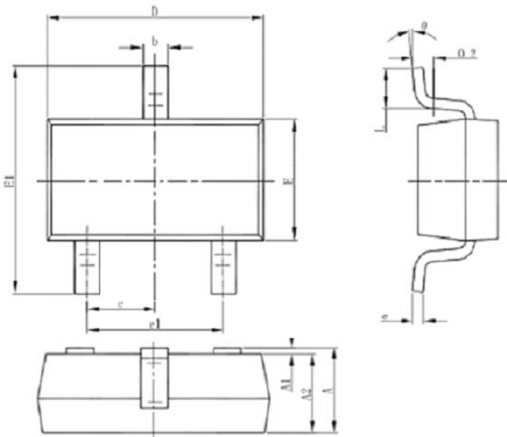
SOT-23-3
