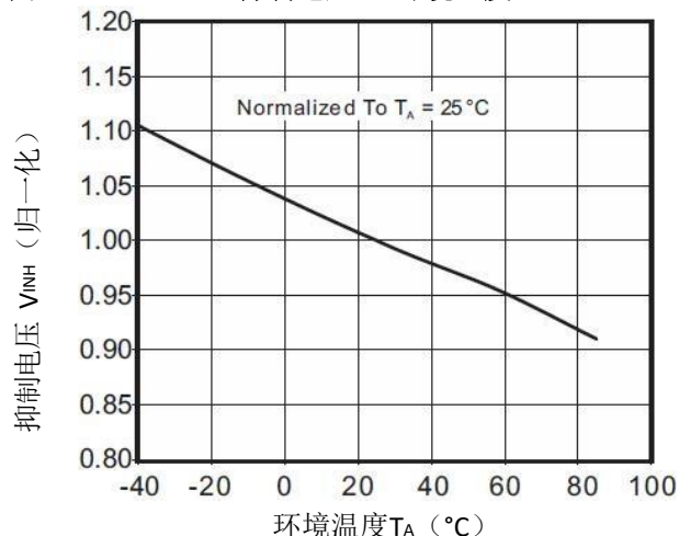
图8 抑制电压 vs 环境温度
