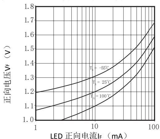
图1 LED 正向电压 vs 正向电流
