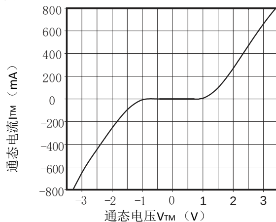
图2 通态电压 vs 通态电流
