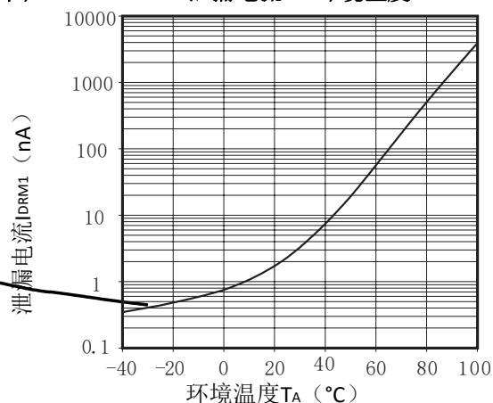
图6 泄漏电流 vs 环境温度
