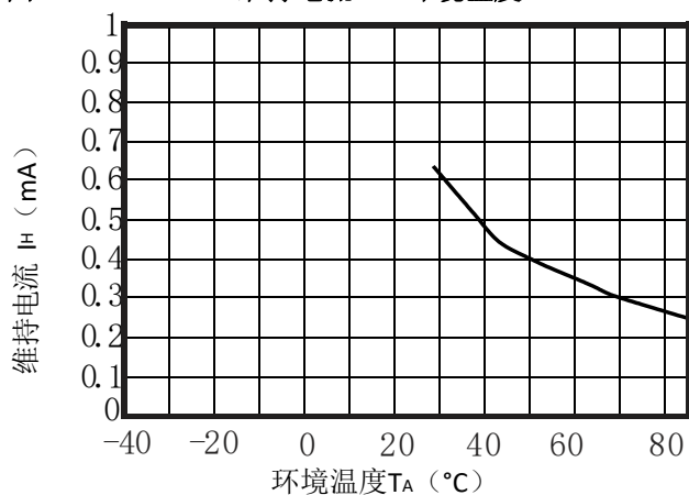
图5 维持电流 vs 环境温度
