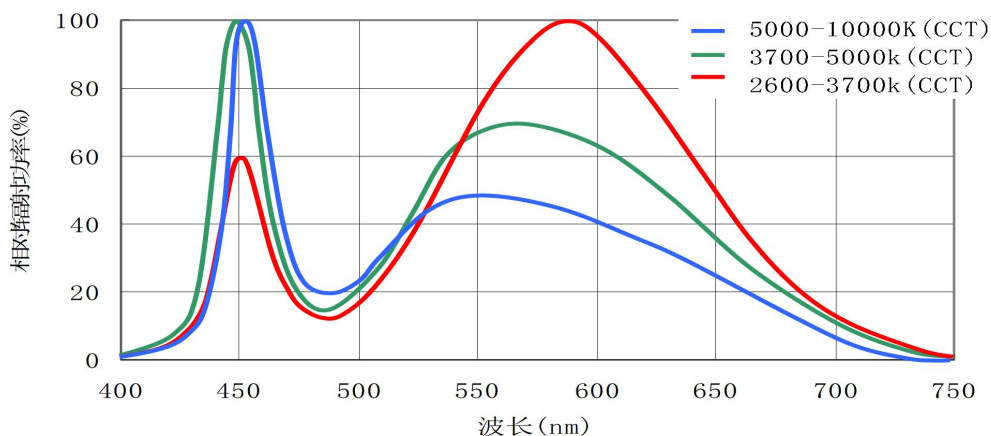
相对光谱功率分布
