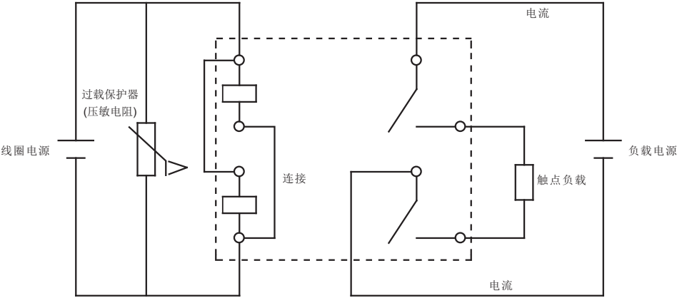
线圈并联接线图（图2）
