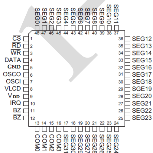
LQFP48
