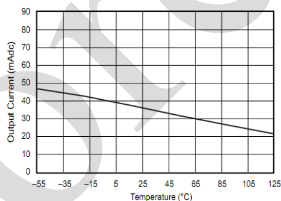
图 10: 源电流限制
