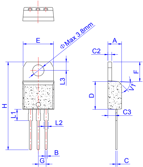
TO-220A Ins
