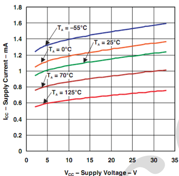
图 1: 电源电流随电源电压变化
