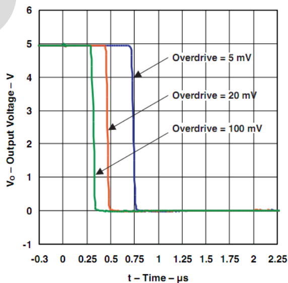
图 4: 过载负载转换响应时间
