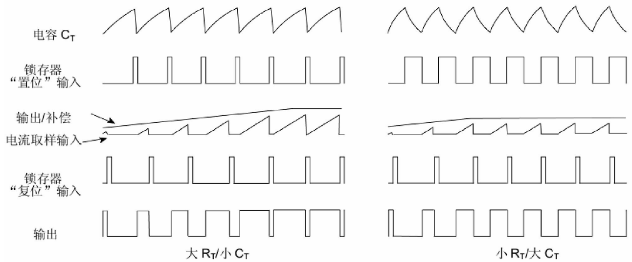
图 18. 时序图
