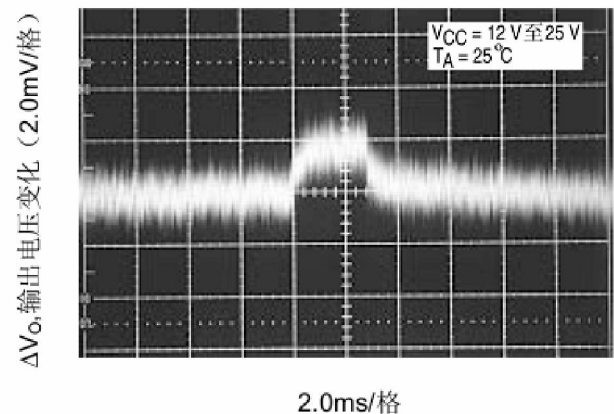
图 12. 参考电源调整率
