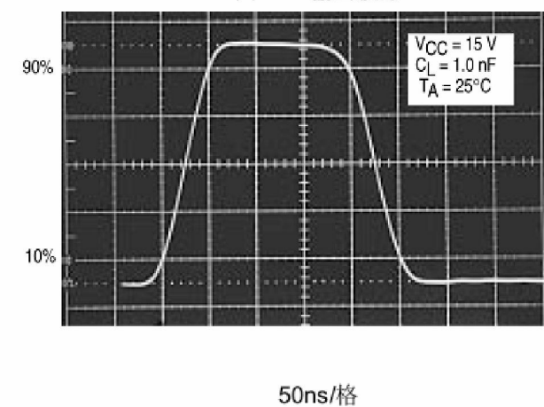
图 14. 输出波形
