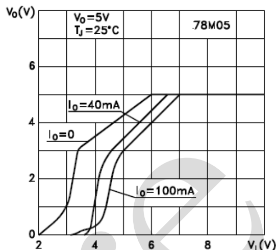
压差曲线
