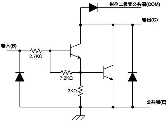
ULN2003A 单路驱动电路原理图
