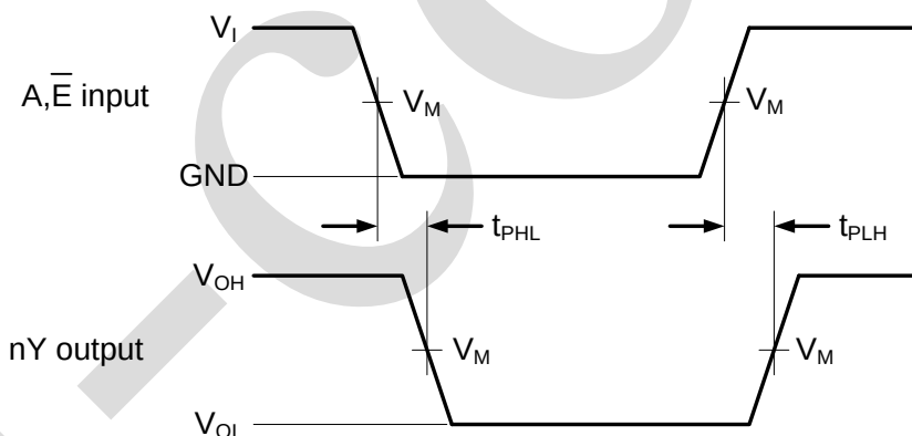
图3 输入A, \bar{E} 到输出Y的输延迟及输出转换时间
