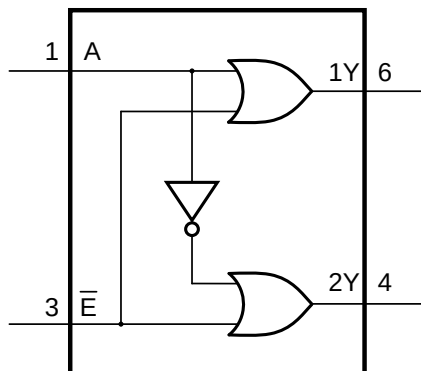
图 1 逻辑符号
