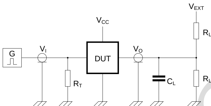
图2 测试开关时间的测试电路
