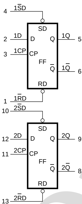
图 4 功能框图
