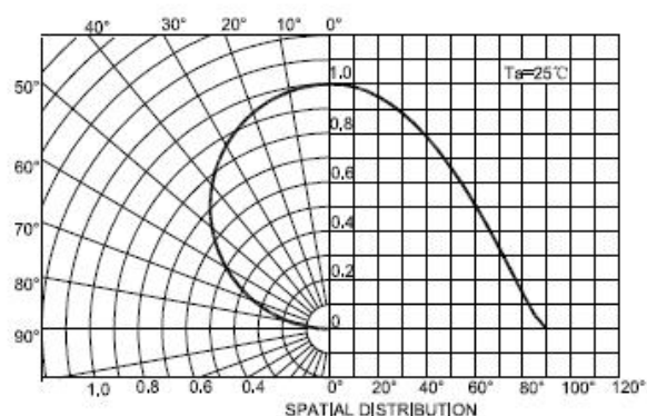
Radiation diagram 辐射图特性曲线
