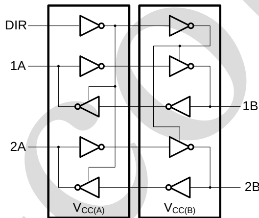
图 2 逻辑框图
