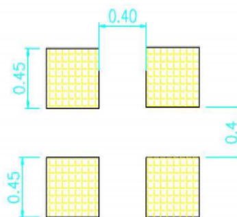
建议焊盘尺寸
