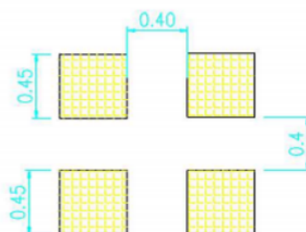
建议焊盘尺寸
