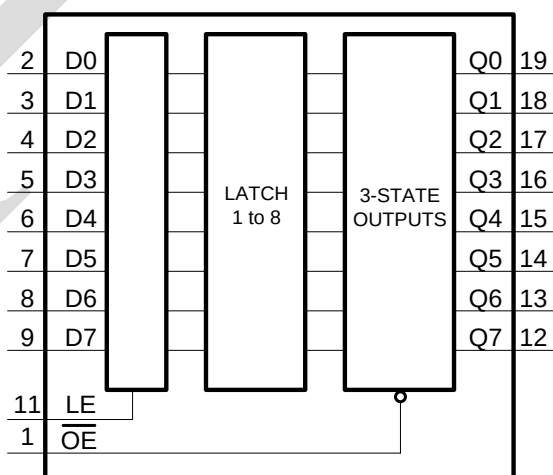
图 3 功能框图
